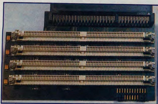
Η Εξχωριστή κάρτα για την αύξηση μνήμης του συστήματός σας. Τα slots της μπορούν να φιλοξενήσουν SIMMS των 4, 8, 16, 32MB των 70ns χωρίς κανένα πρόβλημα.
