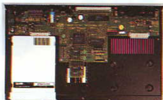
L'interno della macchina mostra una lunga e attenta progettazione. Il lungo chip poco sopra al connettore bianco per le espansioni è il microprocessore Z80B, mentre il chip quadrato al centro della piastra è l'ASIC - una unità che connette tutte le altre parti della macchina.
