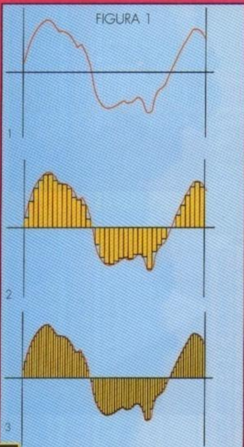
La forma d'onda del diagramma 1 viene riprodotta con poca precisione a una frequenza di campionamento bassa (2) e molto meglio con una frequenza più alta (3)
