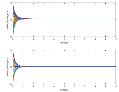
Figura 5. Velocità dello stormo.
