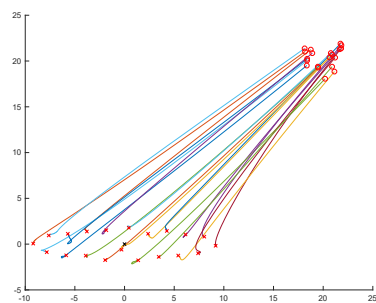
Figura 8. Swarm in una ellisse.
