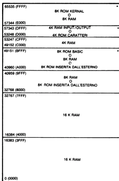
Figura 8.2 Mappa della Memoria
