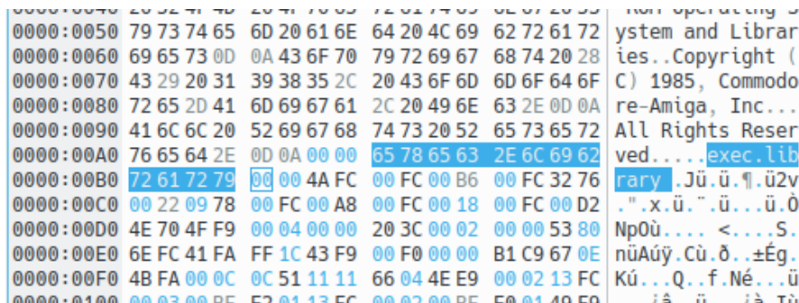
Figura 1 - Editor esadecimale che mostra la rappresentazione ASCII del codice binario.
