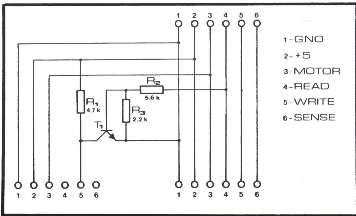
Rys. 1. Schemat elektryczny układu
