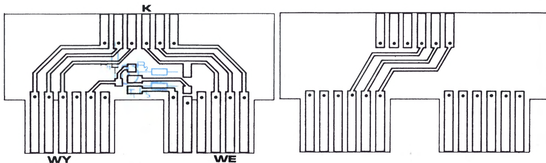
Rys. 2a i b. Ustawienie elementów na płytce
