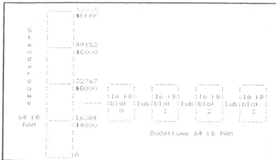
2. Organizacja pamięci mikrokomputera Atari 130XE
