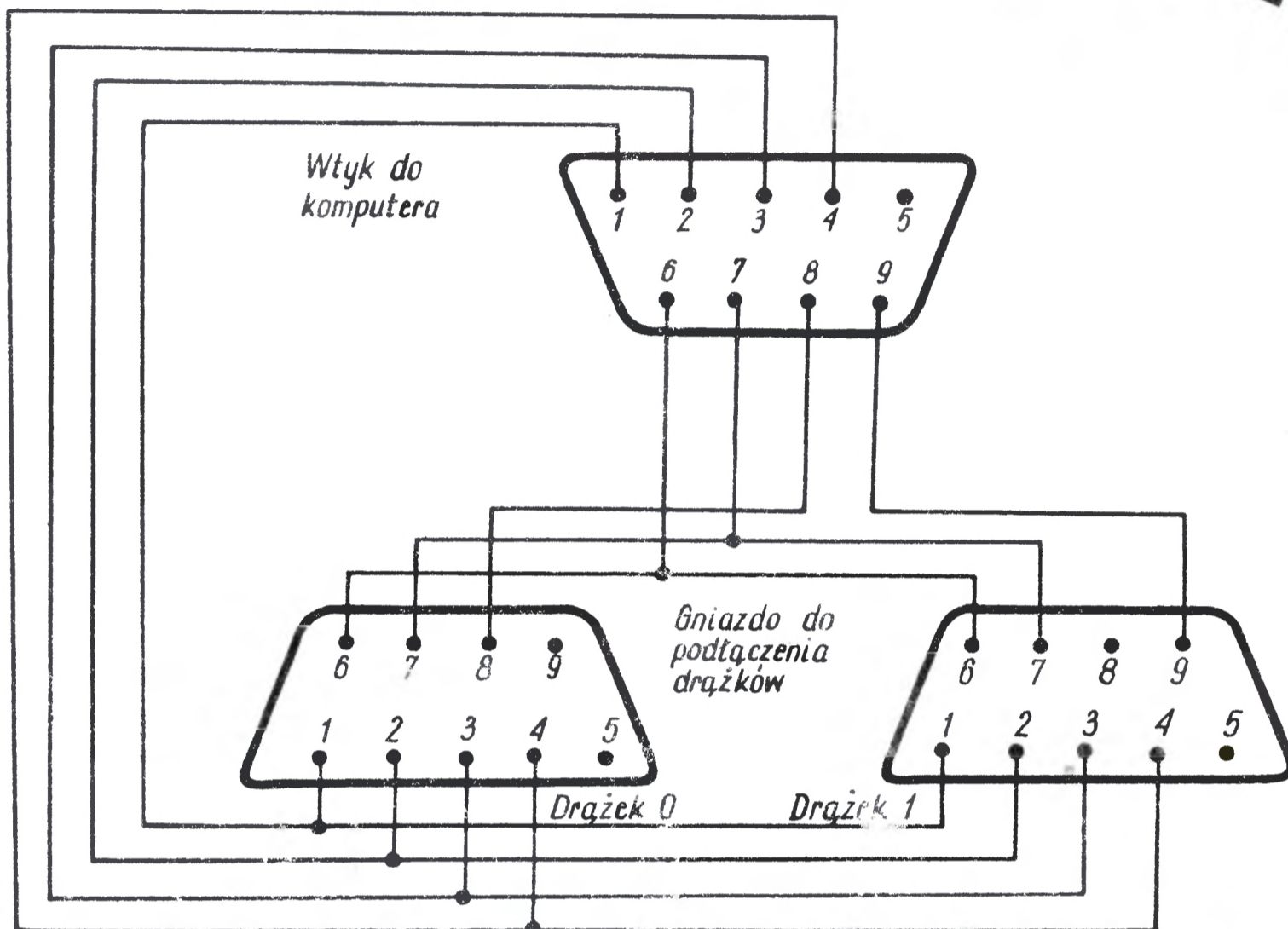
Rys.1. Schemat podłączenia dwóch drążków sterowych do mikrokomputera Amstrad-Schneider (widok gniazd i wtyczki od strony połączeń lutowniczych).
