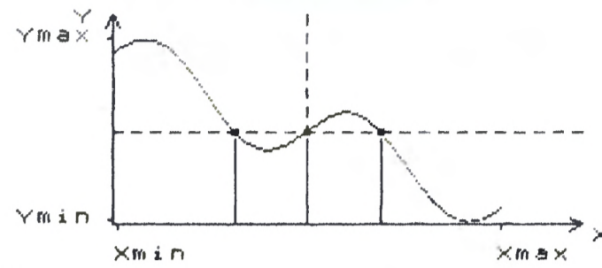
PRZEBIEG FUNKCJI y = \sin x - x/3
