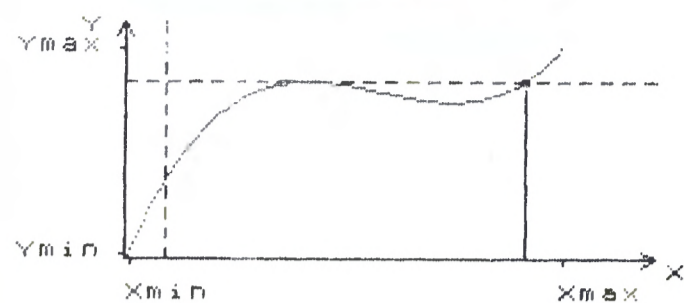
PRZEBIEG FUNKCJI y = x^3 + 9x^2 + 24x - 20
