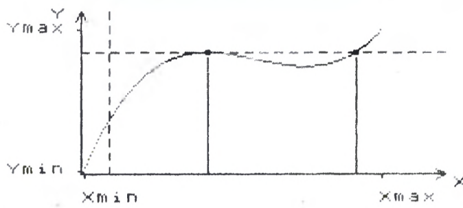
PRZEBIEG FUNKCJI y = x^3 + 9x^2 + 24x - 20
