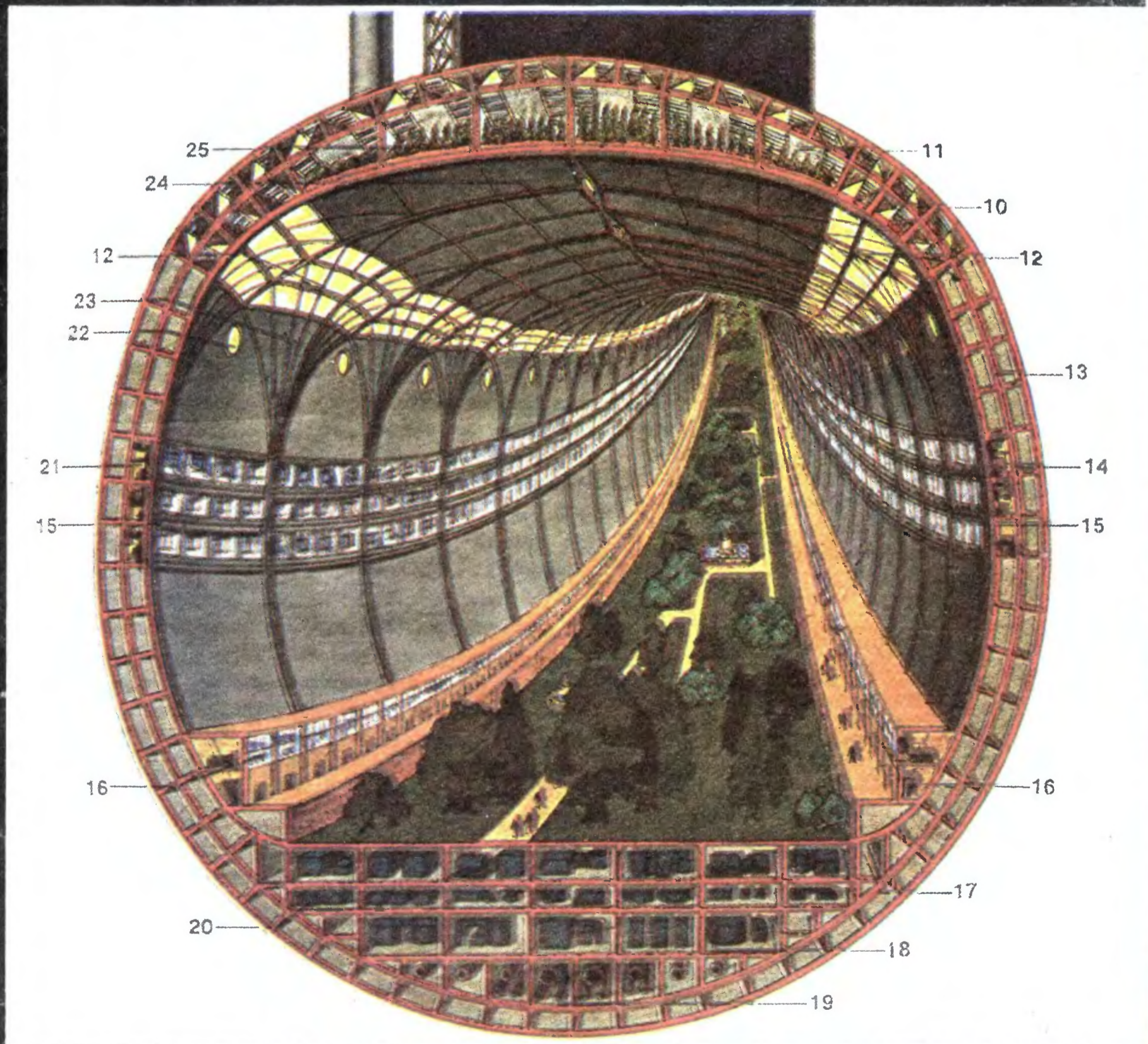
Przekrój poprzeczny kosmicznego miasta typu toroidalnego. 10. Lustra oświetlające okna głównej przestrzeni życiowej miasta. 11. Lustra oświetlające strefę rolniczą. 12. Okna głównej przestrzeni życiowej miasta. 13. Bloki konstrukcyjne toroidu. 14. Aparatura w wewnętrznych sekcjach ścian. 15. Balkony. 16. Główną strefa mieszkalna miasta — z kawiarniami i sklepami na parterze. 17. Schrony awaryjne. 18. Strefa przemysłowa. 19. Podstawowe rurociągi i kable systemu zasilania i łączności. 20. Magazyny. 21. Zaplecze systemu sterowania. 22. Sztuczne oświetlenie. 23. Konstrukcje szkieletu wewnętrznego. 24. Dach (znajduje się w odległości 113 metrów od „ziemi”). 25. Strefa rolnicza.
