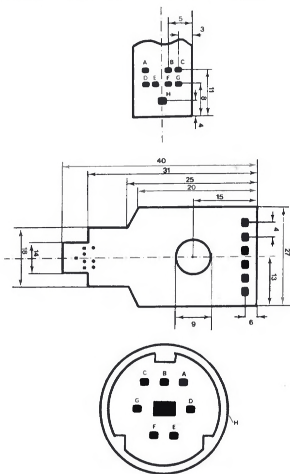
Rys. 3 Płytką złącza pośredniego (widok od strony druku).
