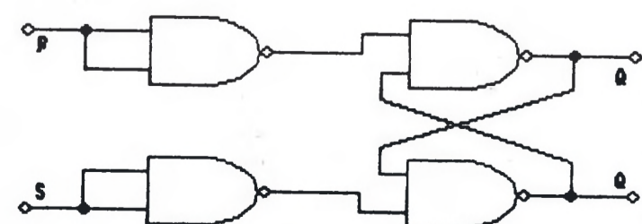
Rys.9 — Przerzutnik RS
