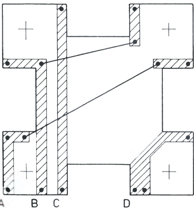
Płytki drukowana dodatkowych klawiszy (rysunek bez skali) — widok od strony druku. Dwie ciągłe linie — zwory: A, B, C i D — wyjścia.
