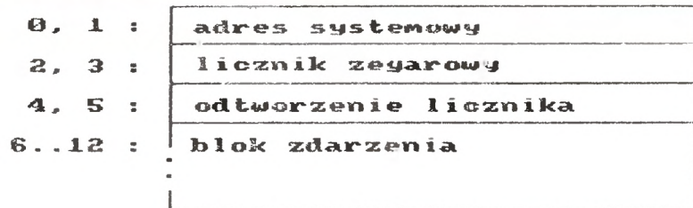
Rys. 2. Blok kolejki zwykłego zegara.
