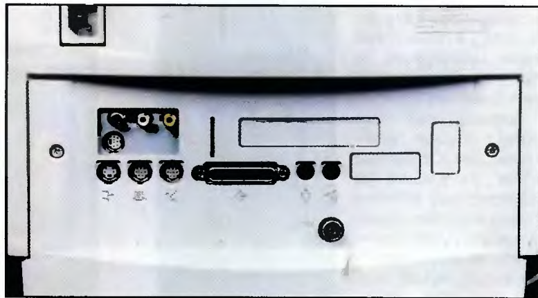
Złącza na tylnaj ścianie komputera.
