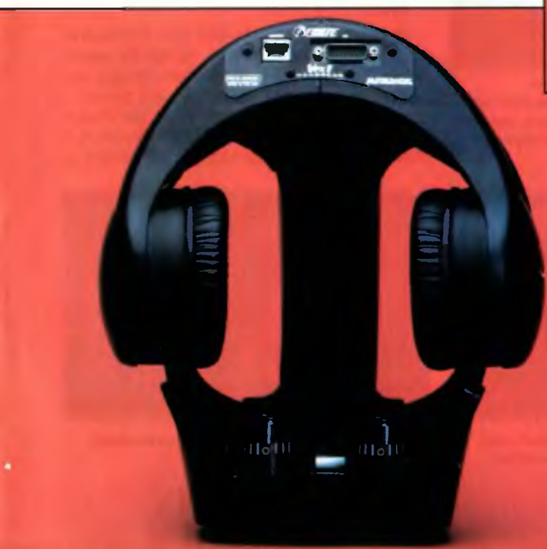
VFX1 „od podszewki” – widoczna jest podziałka od regulacji ostrości oraz dwa gniazda: 26-pinowe na kabel łączący z komputerem oraz ACCESS.bus na CyberPuck-a.
