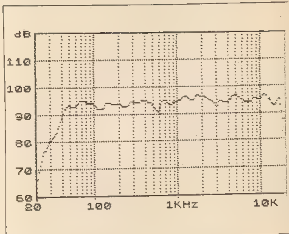
Skica 14: Frekvenčna karakteristika odziva zvočnika
