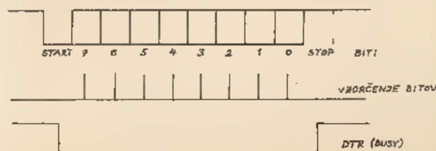
Časovni diagram prenosa podatkov pri vmesniku RS232
