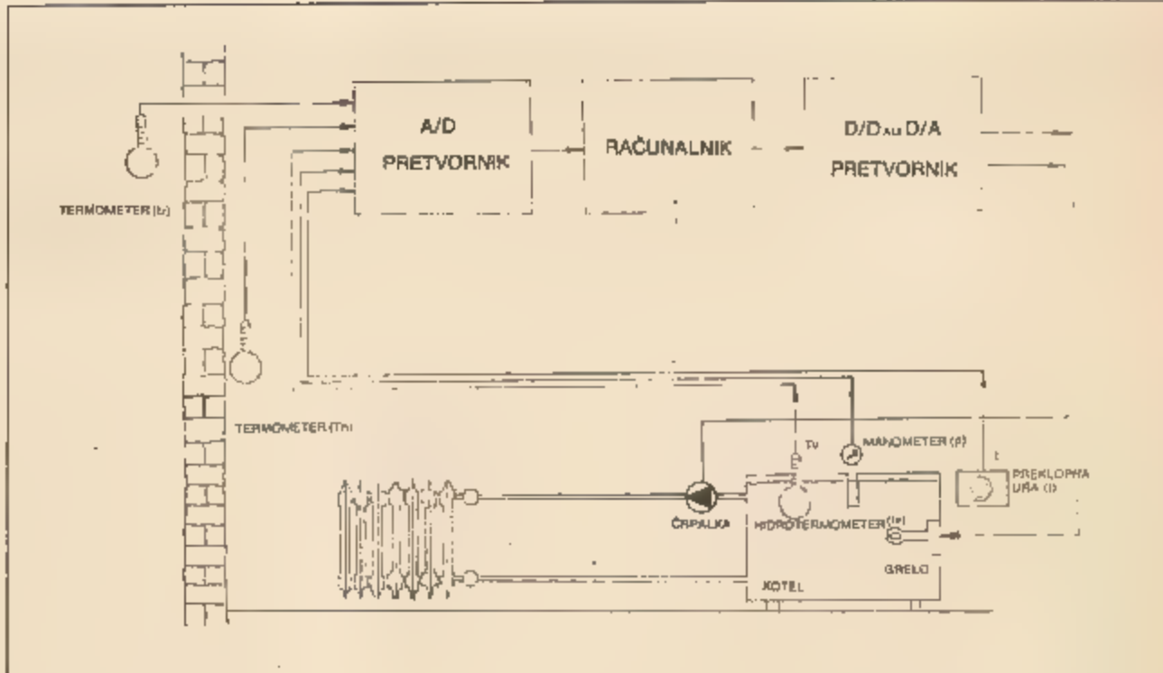
Skica 18: Vključitev računalnika v proces centralnega ogrevanja
