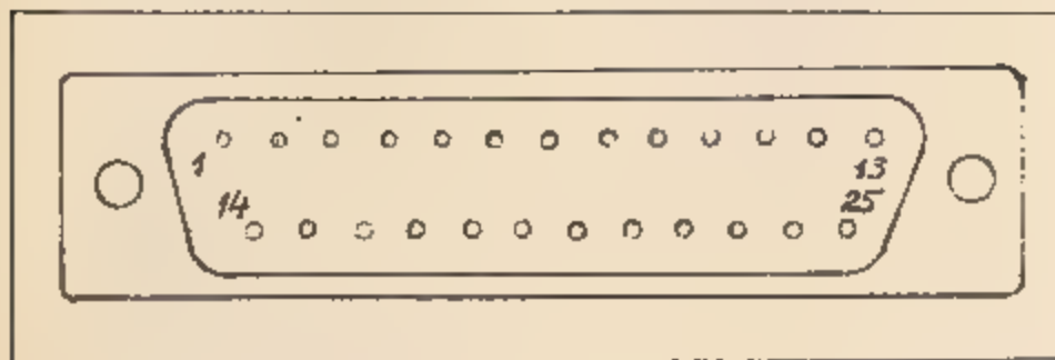
Konektor vmesnika RS232
