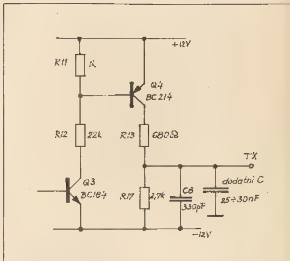
Izhodna stopnja vmesnika RS232 na Interface 1
