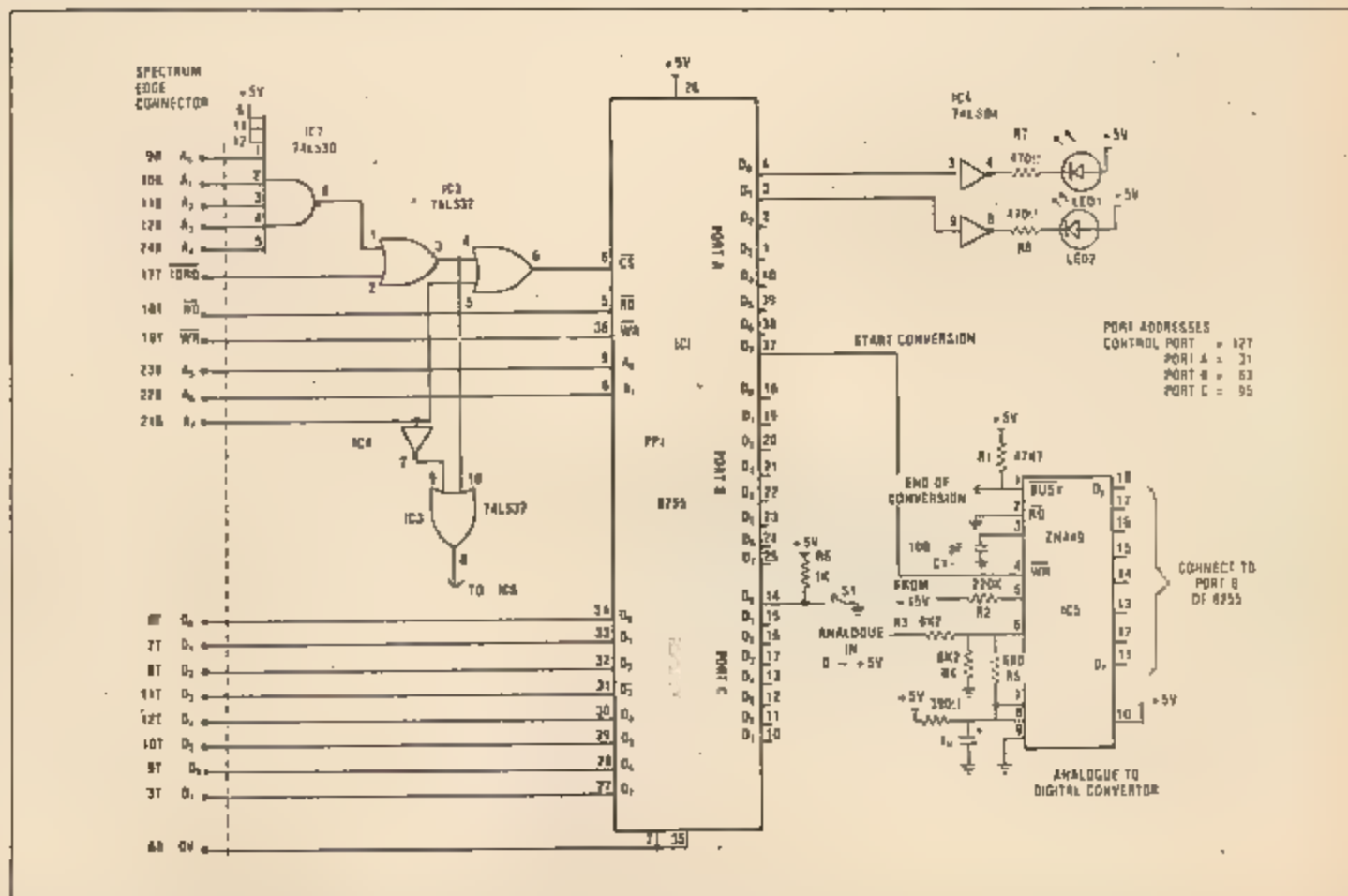
Skica 20: Električna shema analožno-digitalnega pretvornika za mikroročunalnik ZX-Spectrum
