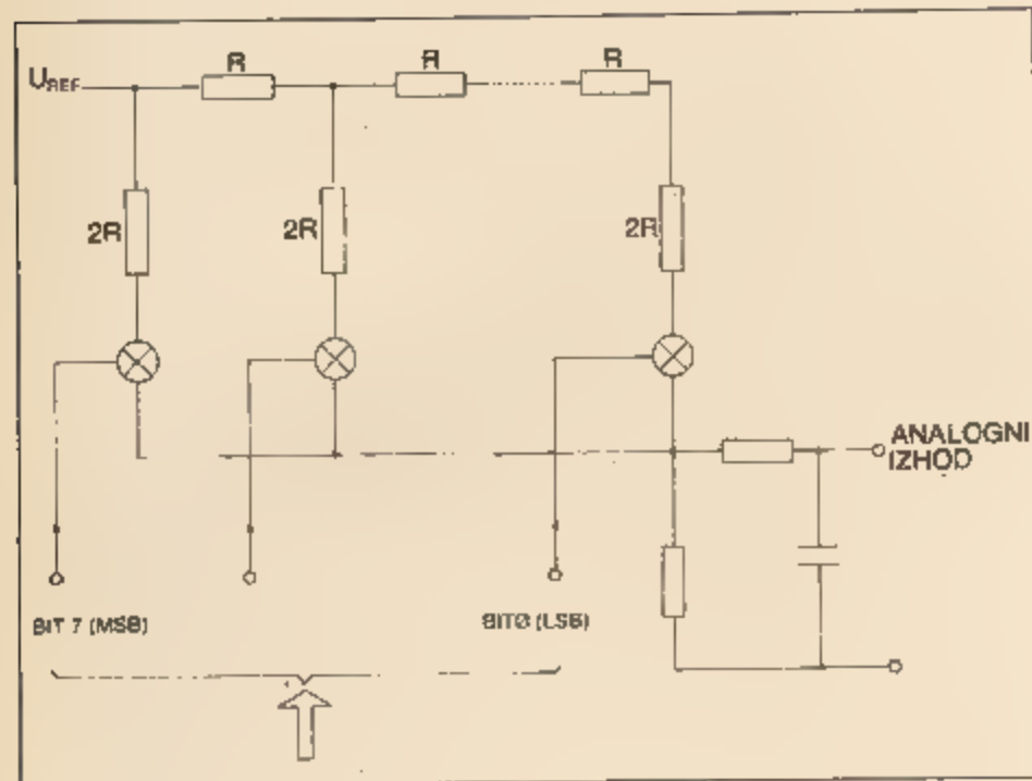
Skica 12: R-2R vezja D/A pretvornika
