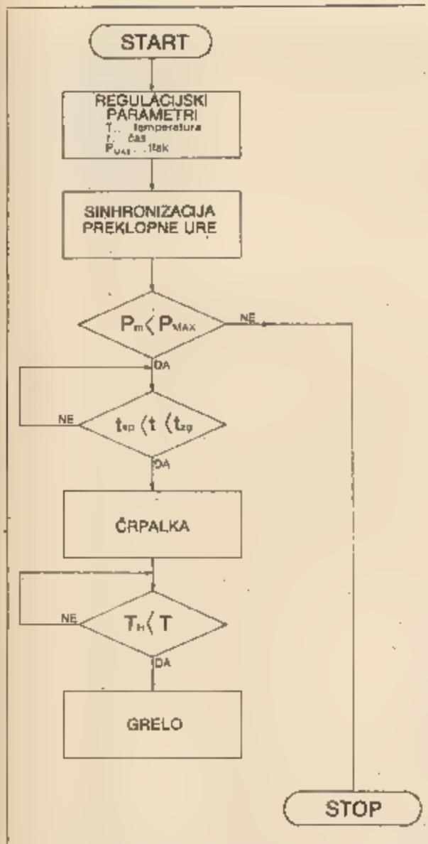
Skica 17: Preprost algoritem regulacije centralnega ogrevanja
