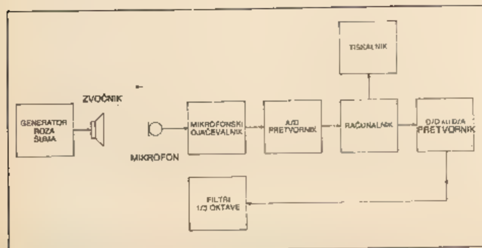
Skica 13: Meritev frekvenčne karakteristike odziva zvočnika
